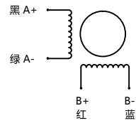
绕组接线图
